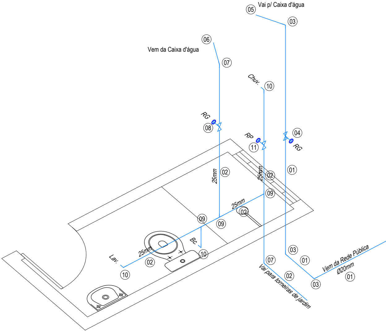
Instalações Hidráulicas - Perspectiva Escala 1 : 25
