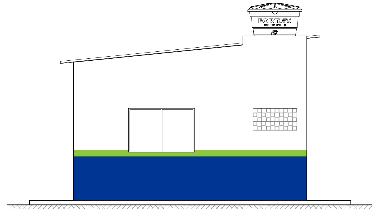
Fachada Lateral Direita Escala 1 : 50
