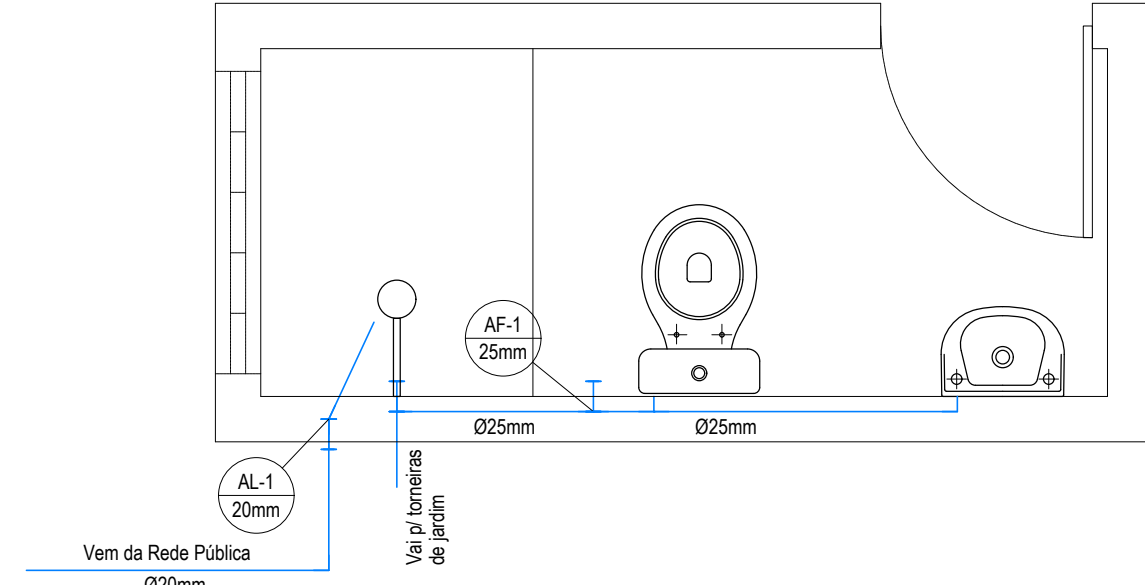
Instalações Hidráulicas - Planta Baixa Escala 1 : 25
