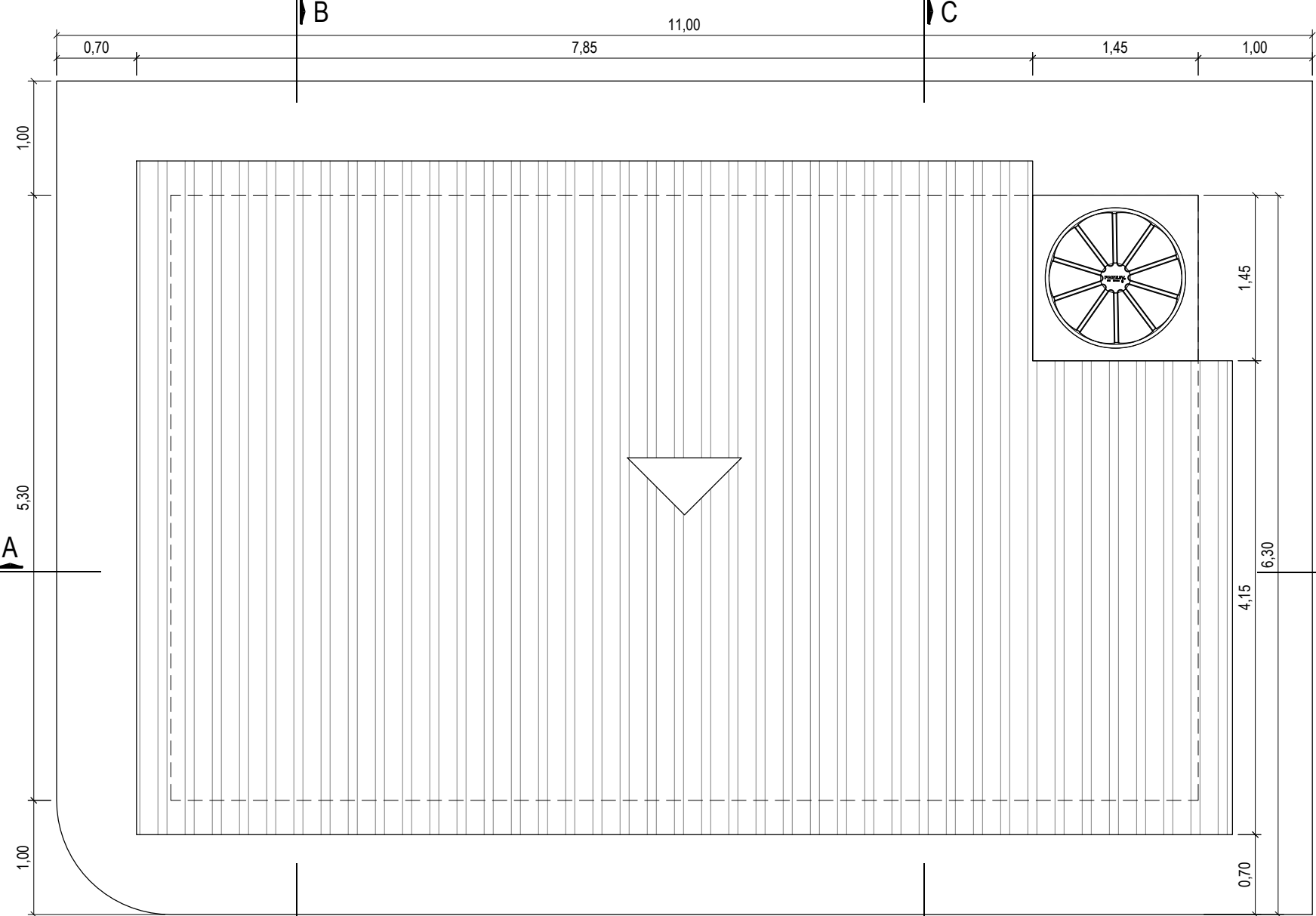
Planta de Coberta Escala 1 : 50
