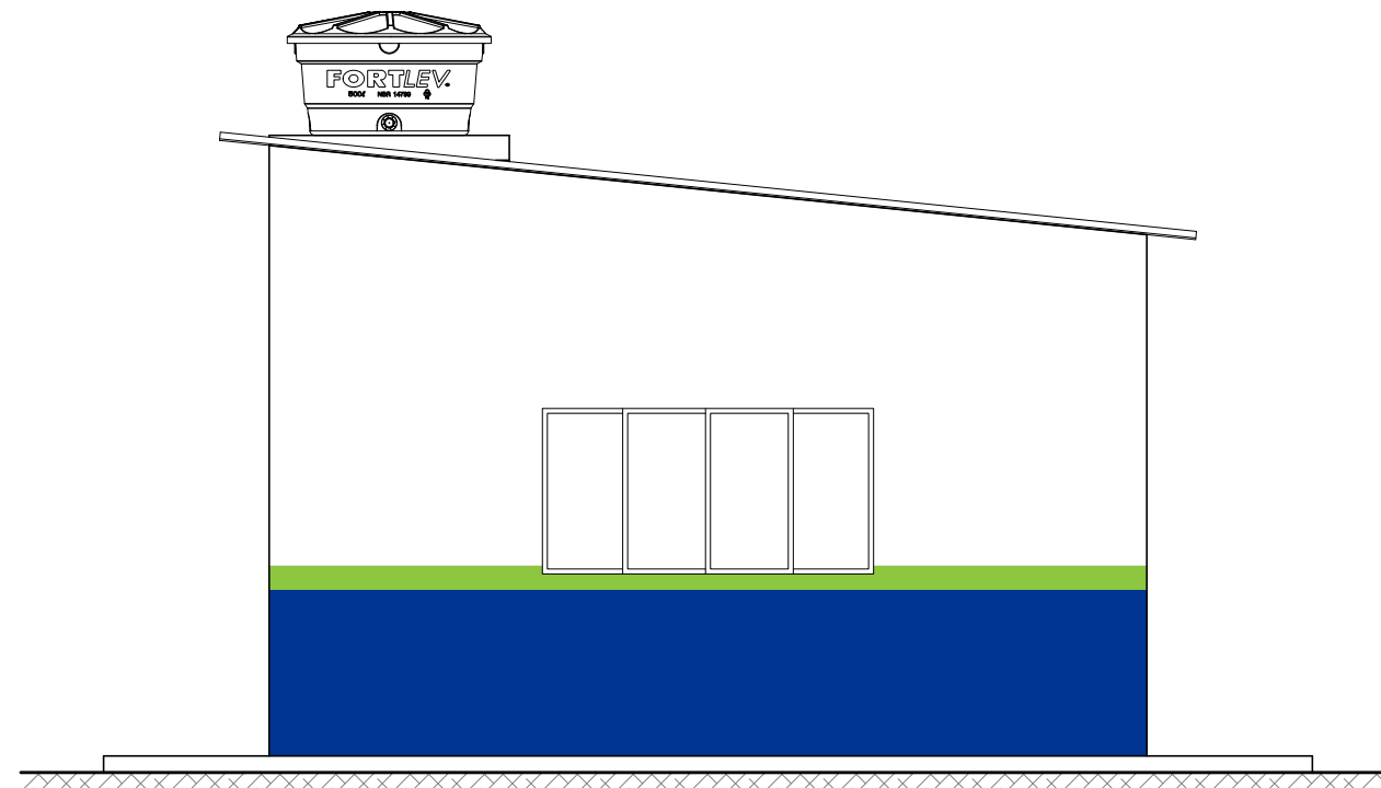
Fachada Lateral Esquerda Escala 1 : 50
